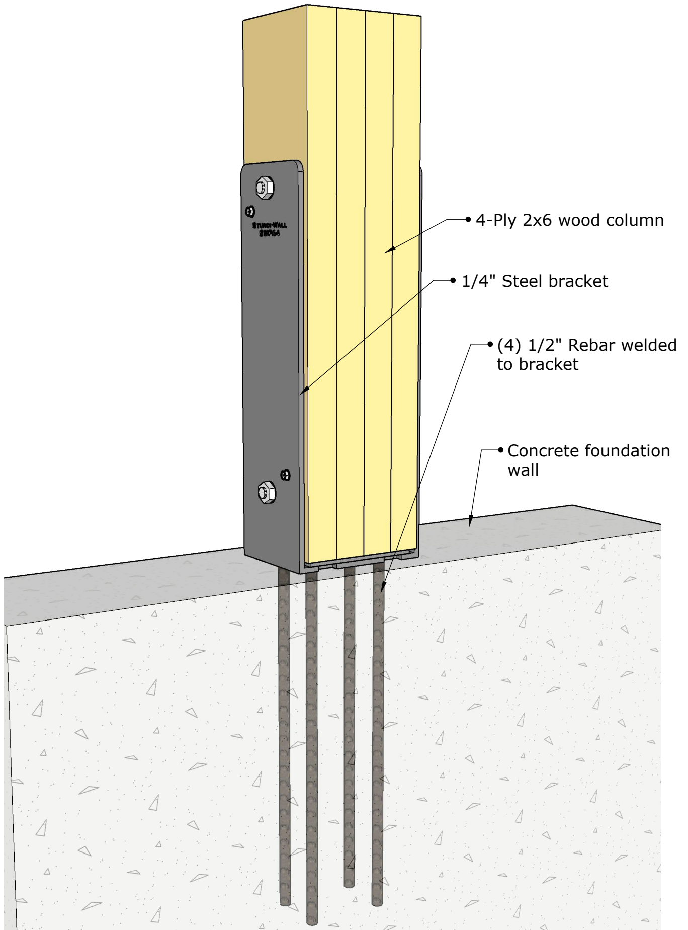
STURDI-WALL PLUS BRACKET SWP64
